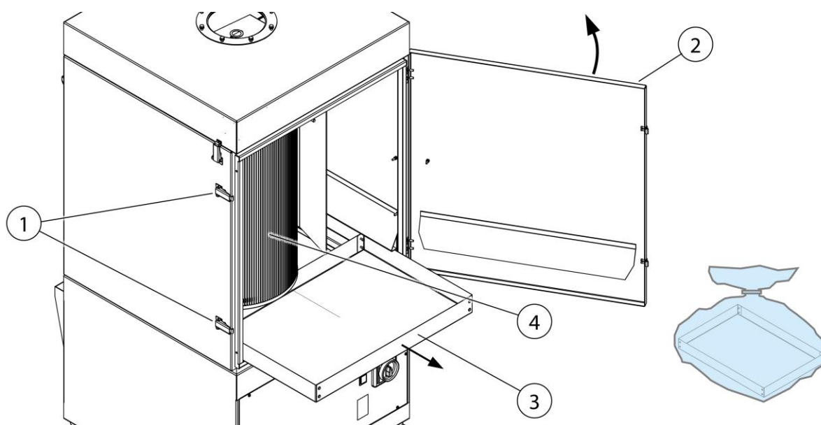
Fig. 7 : Vidange du bac collecteur de poussières
